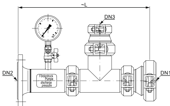
Maßzeichnung: Pumpenverteiler MMP2 dimension drawing: pump manifold MMP2
